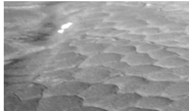
Abb 2: «polygonized tundra»
